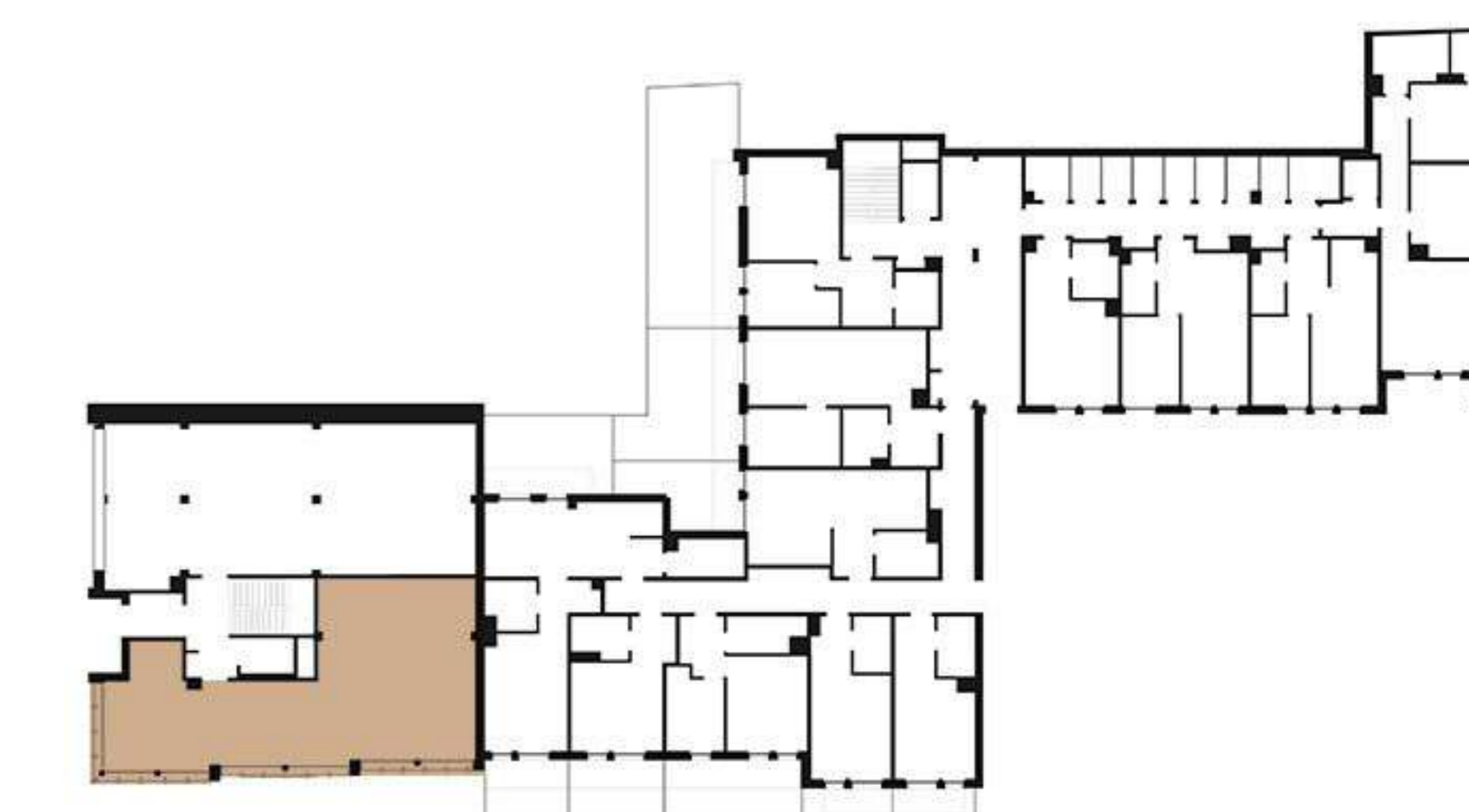
Rzut piętra +1
