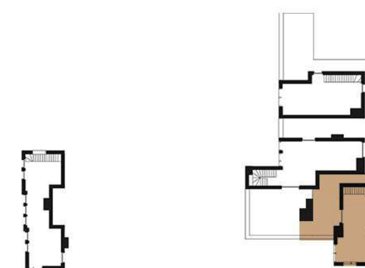
Rzut piętra +5
