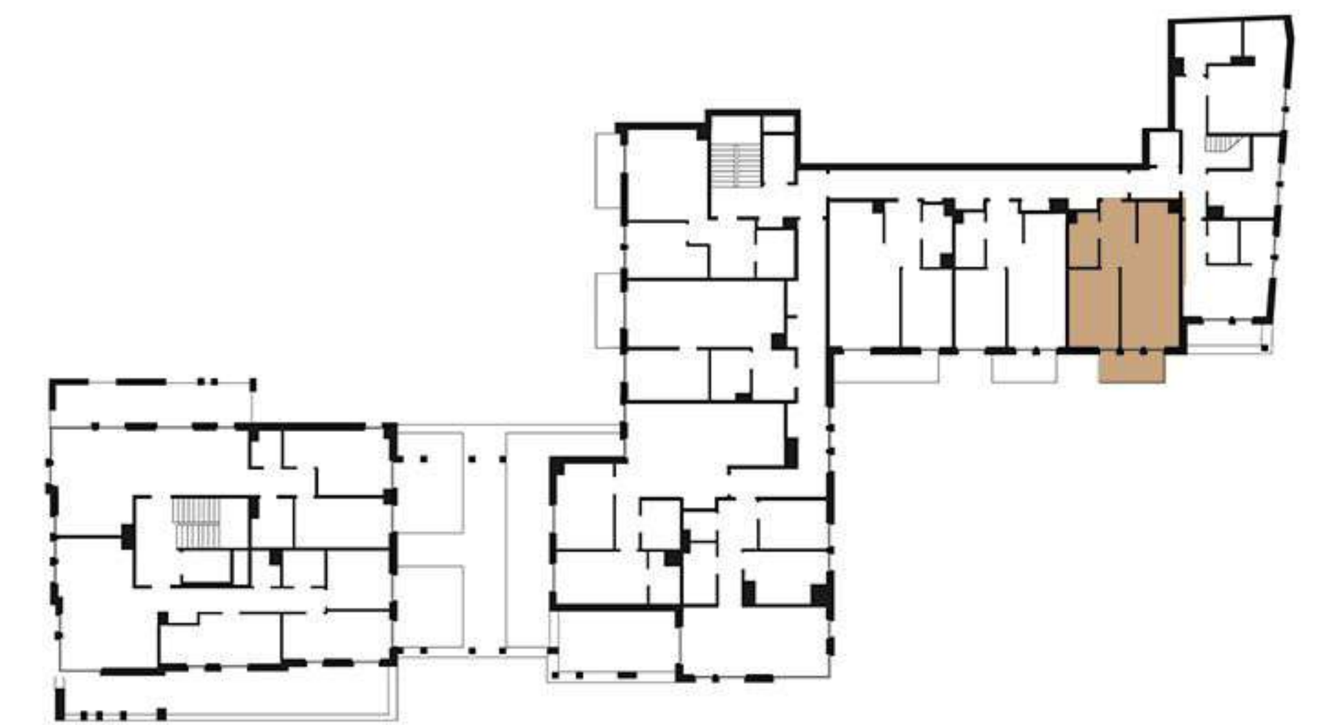
Rzut piętra +2
