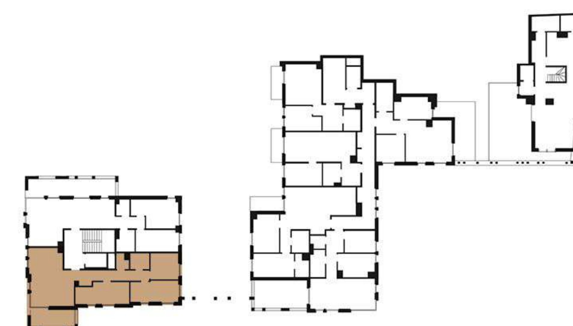
Rzut piętra +3
