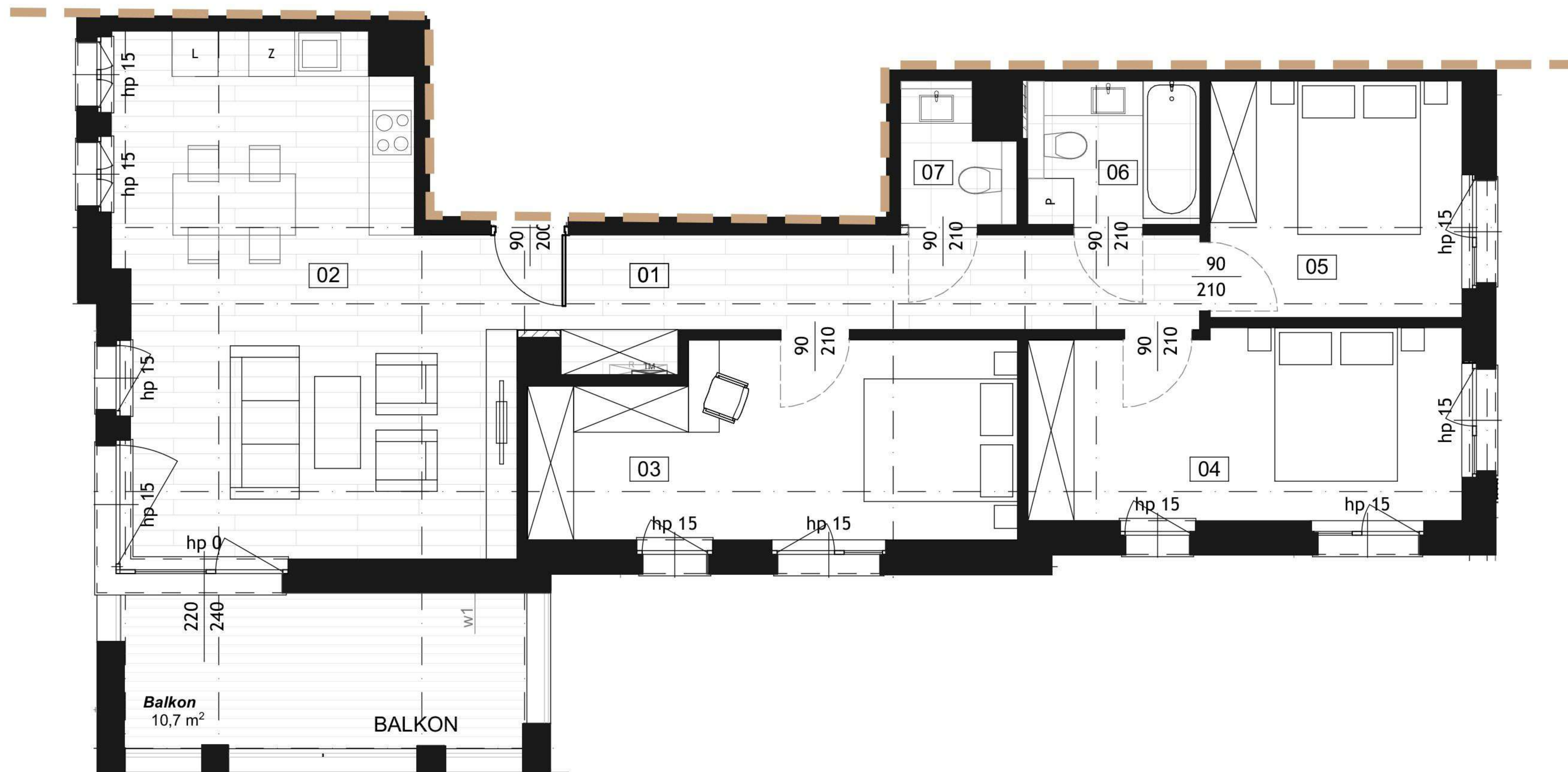
Rzut piętra +3
