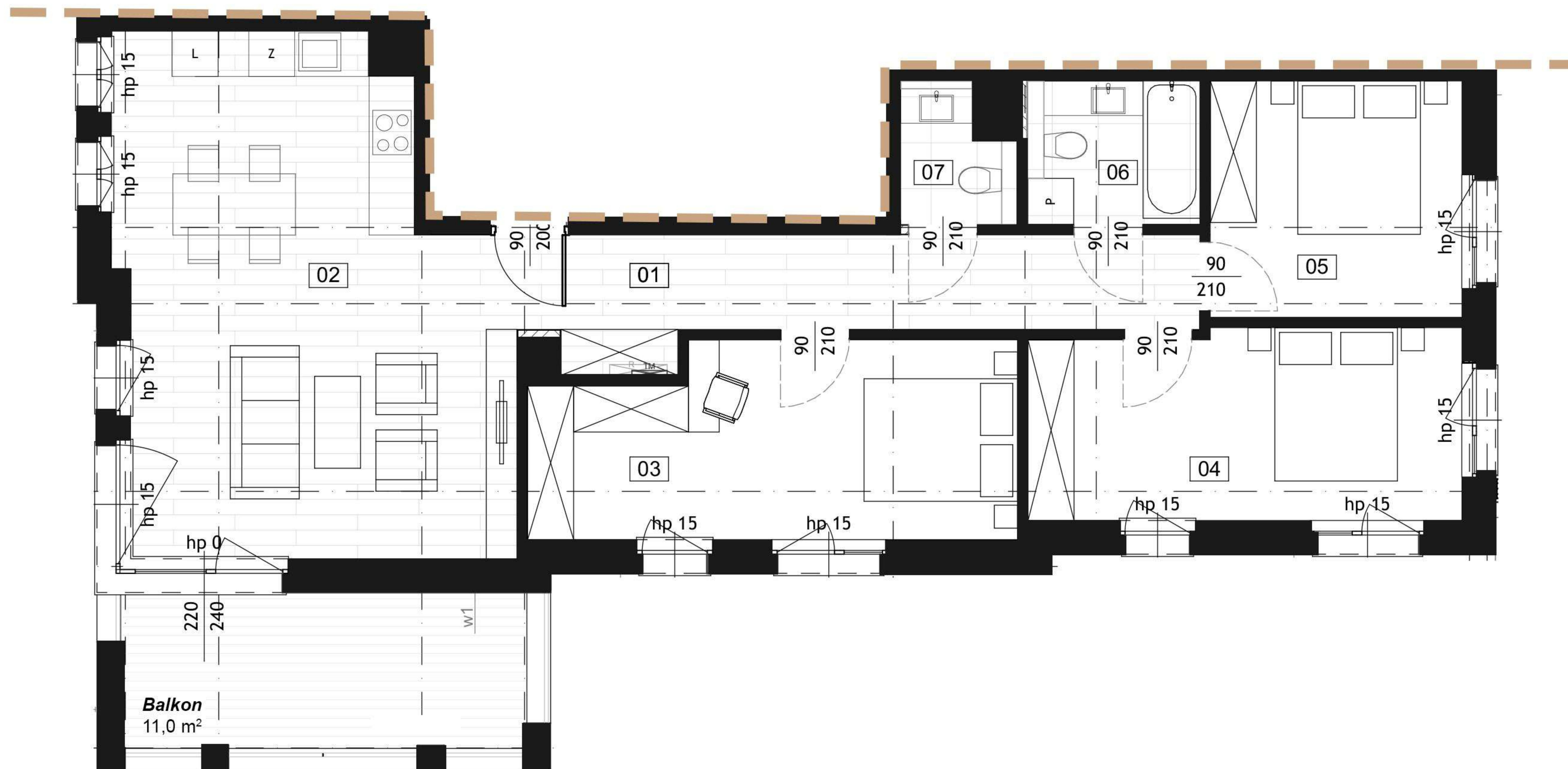
Rzut piętra +3
