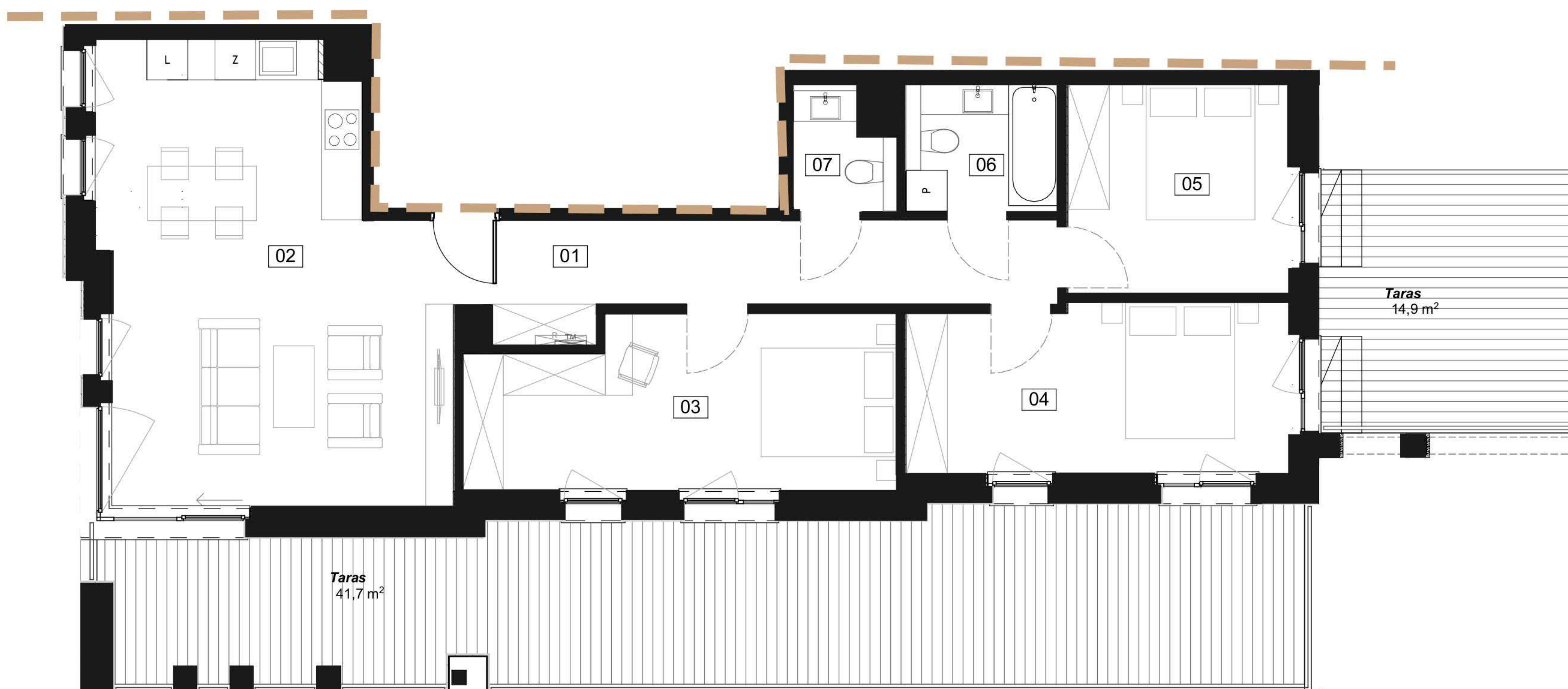
Rzut piętra +2
